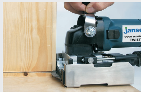
Fitting door frames
